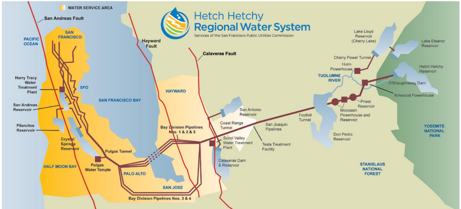
FIGURE 2 - SISTEMA DE AGUA REGIONAL DE HETCH HETCHY
